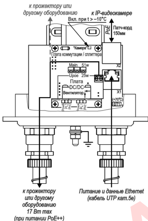
Рисунок 7 – Схема подключения TBK-...-PoE++
