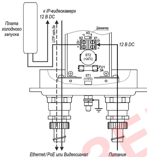
Рисунок 4 – Схема подключения IP-видеокамеры (12VDC)
