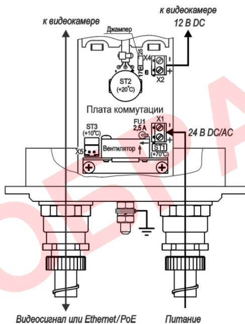
Рисунок 2 – Схема подключения IP-видеокамеры (24VDC/AC)
